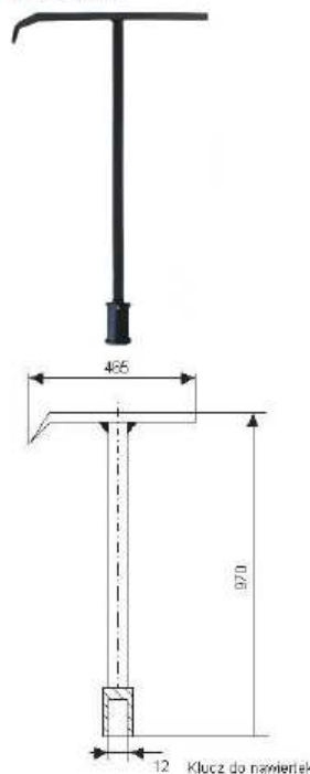
2) Klucz do nawiertek Nr kat. 5025
