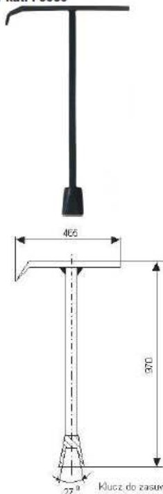
1) Klucz do zasuw i hydrantów Nr kat. : 5030
